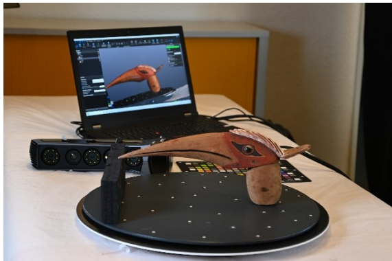
14_Setup für die 3D-Digitalisierung eines Tanzmundstücks aus Papua-Neuguinea mit dem Handscanner im DiViAS-Projekt.
